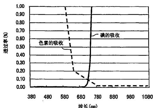
偏光板正交透过光谱
