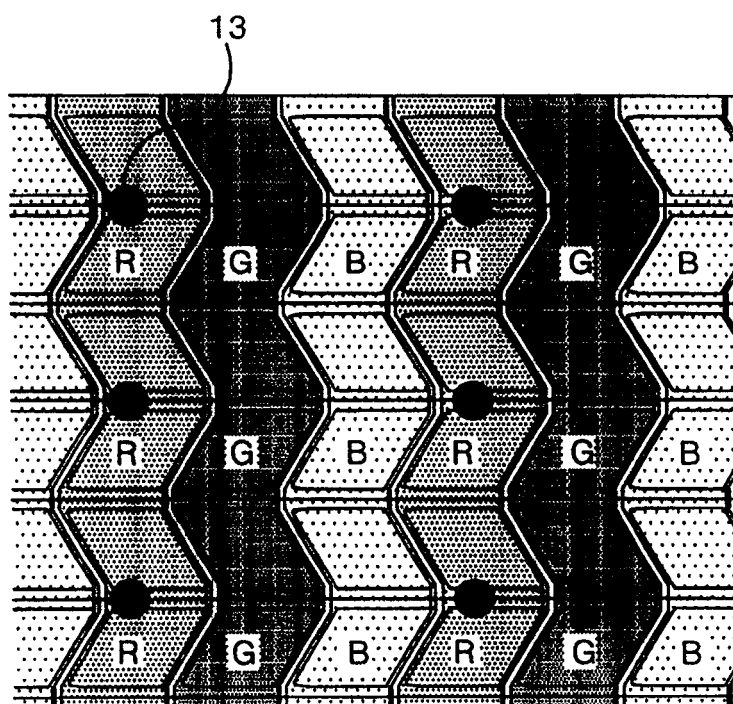
图 1 现有技术
