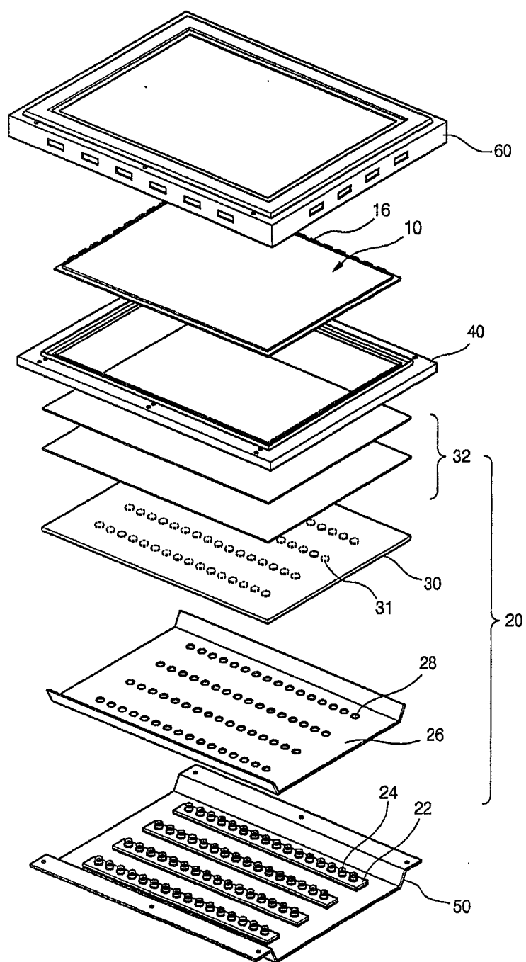
图 1 现有技术
