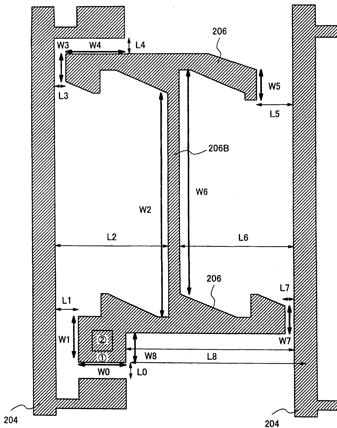
图2B 现有技术
