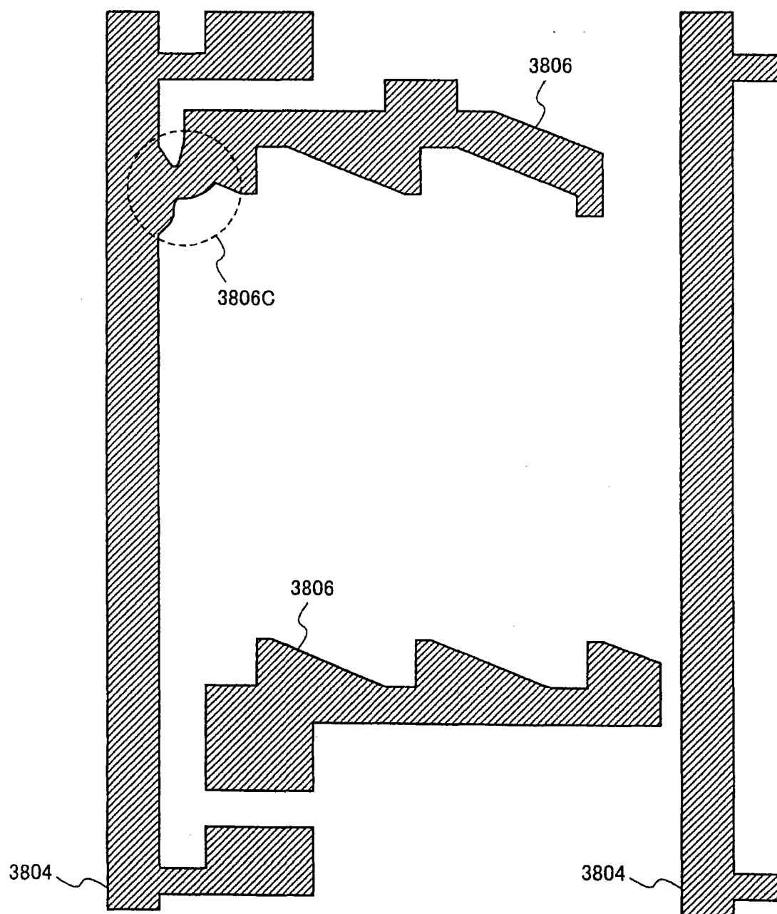
图38B 现有技术
