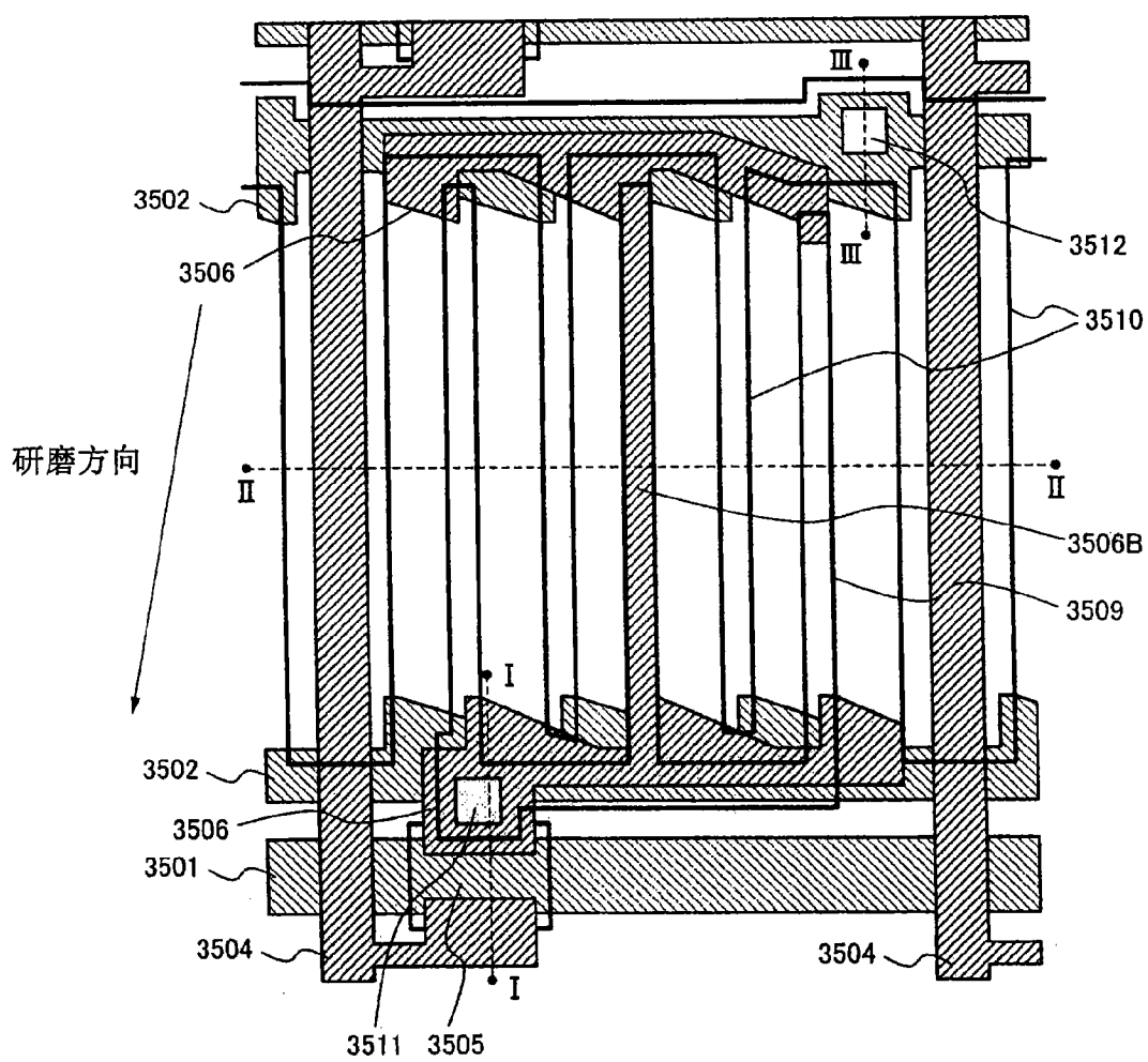
图35A 现有技术
