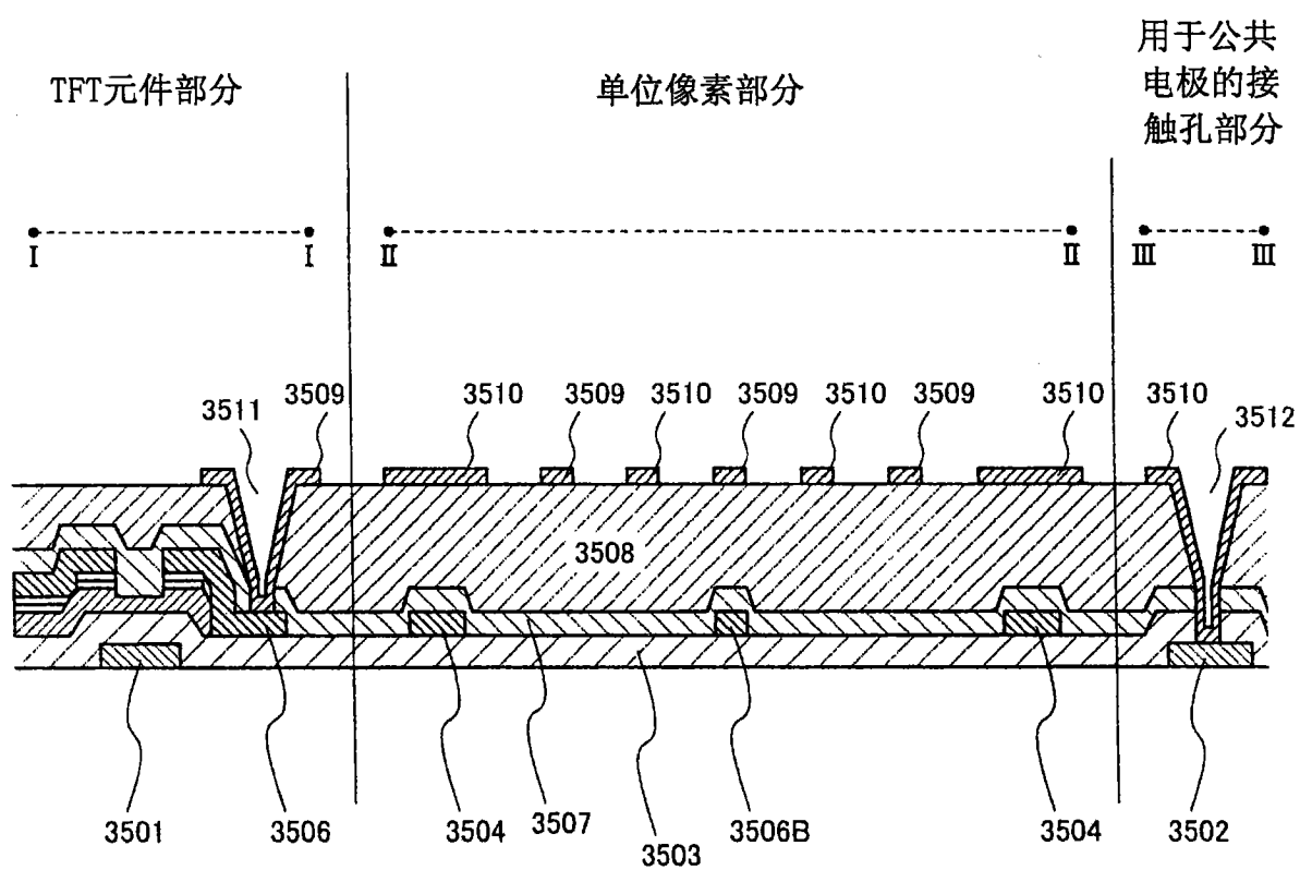
图35B 现有技术
