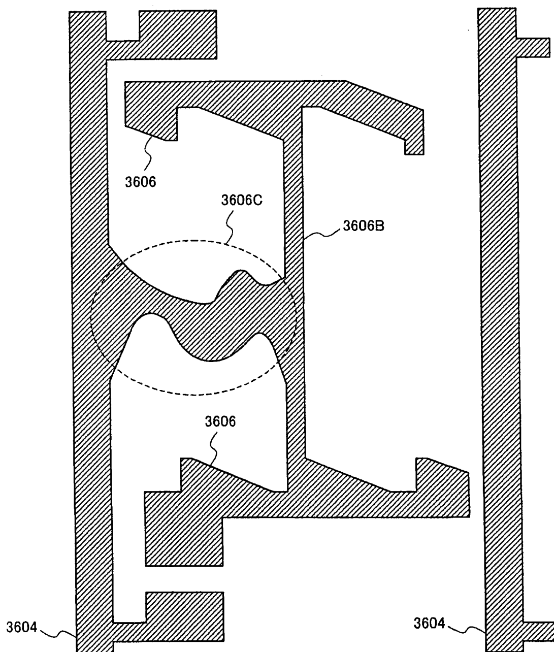
图36B 现有技术
