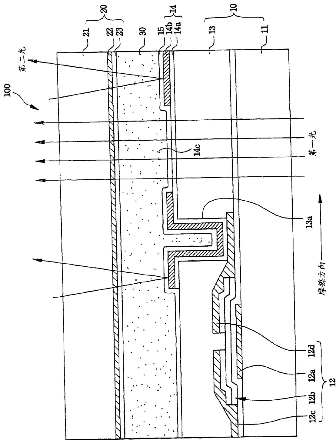
图 1 (现有技术)
