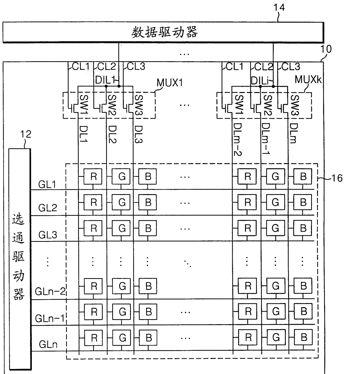
图 1 现有技术
