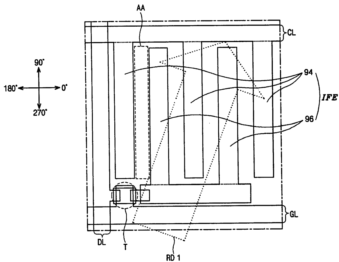
图 4A (现有技术)
