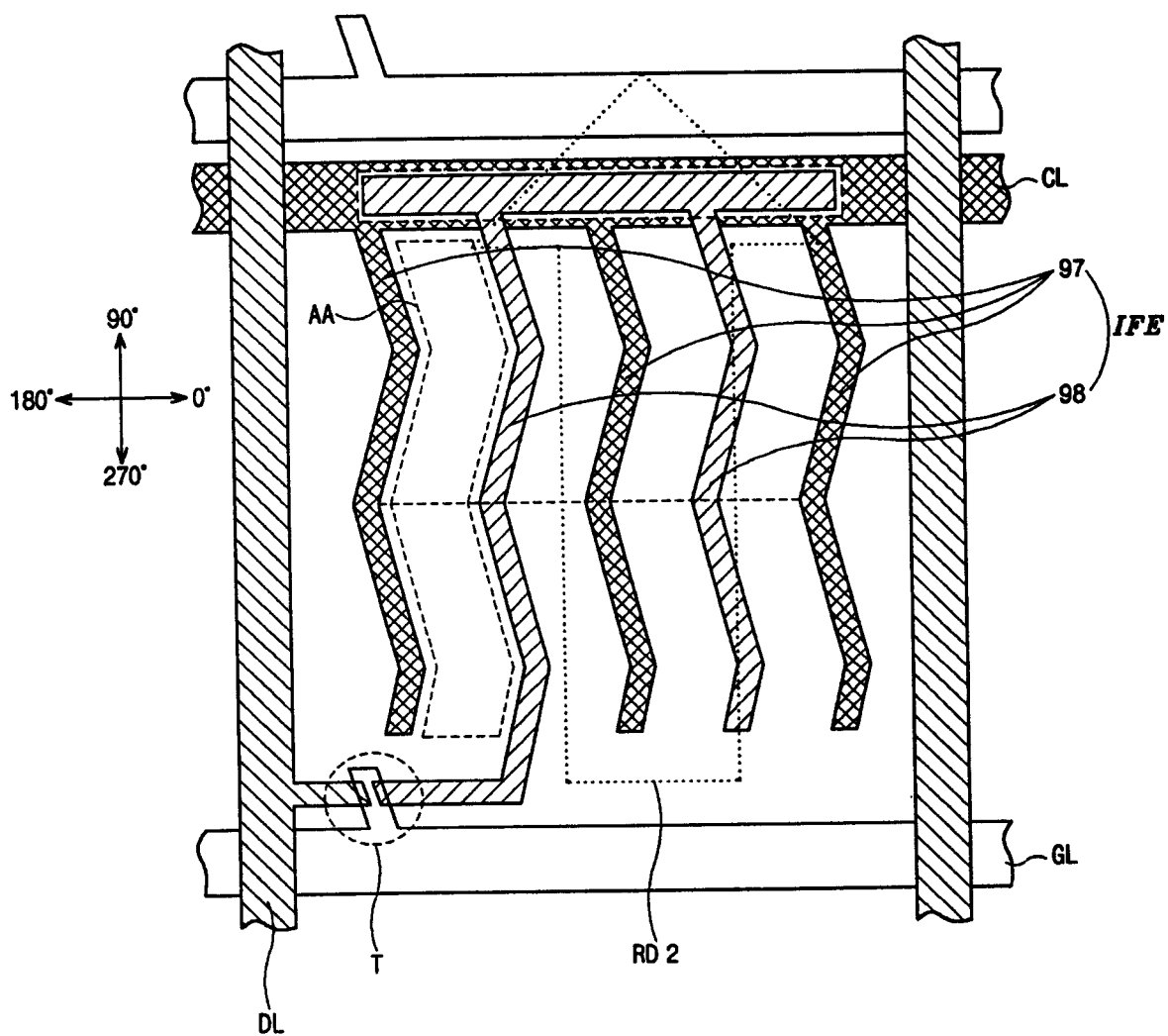
图 4B (现有技术)
