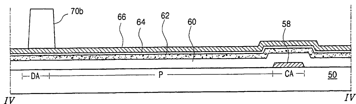
图 4C 现有技术
