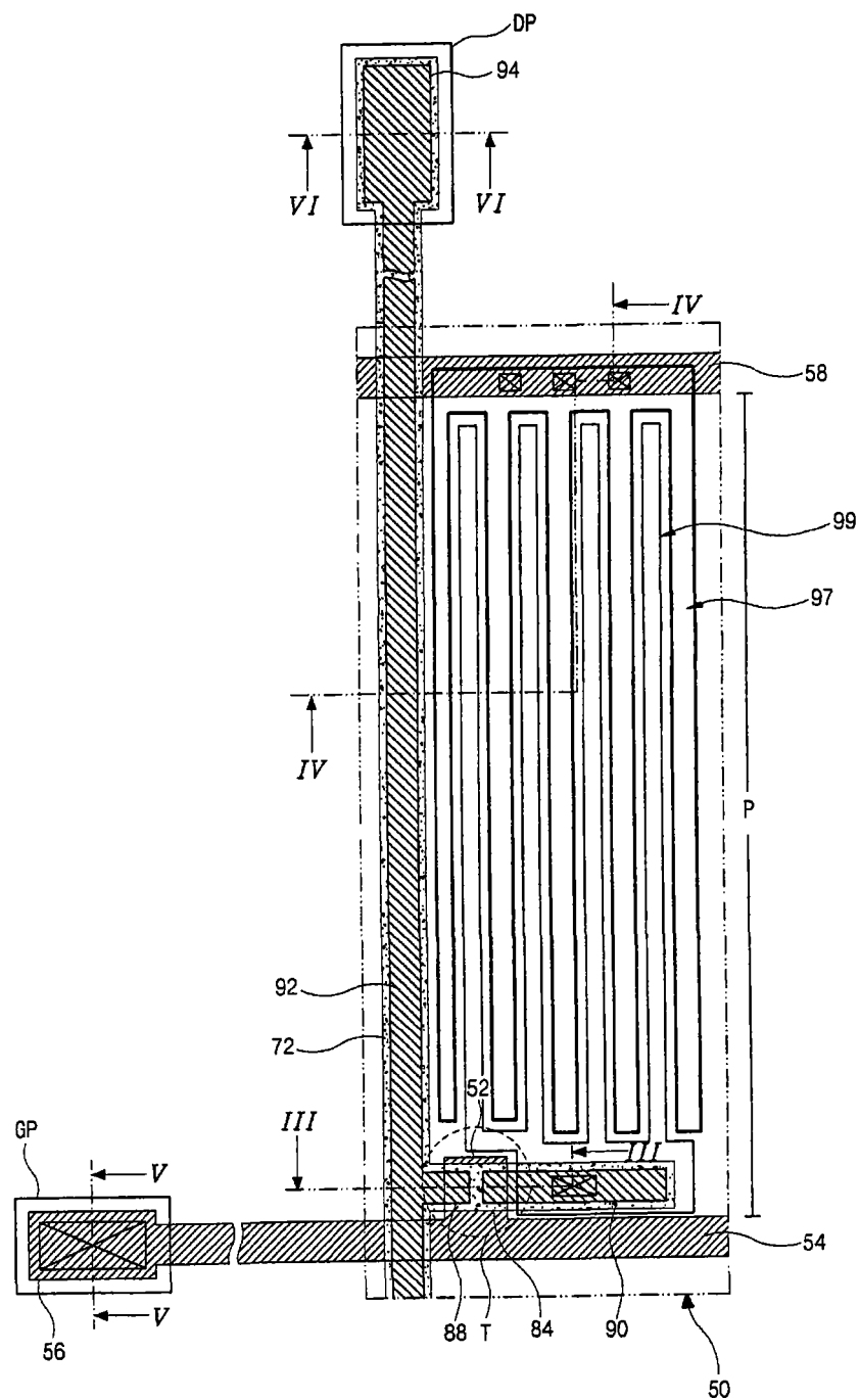
图 2 现有技术
