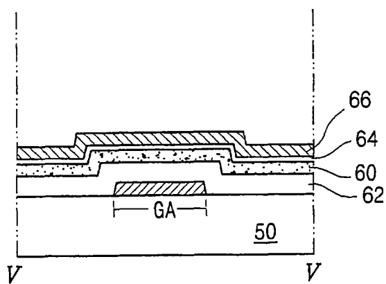
图 5C 现有技术
