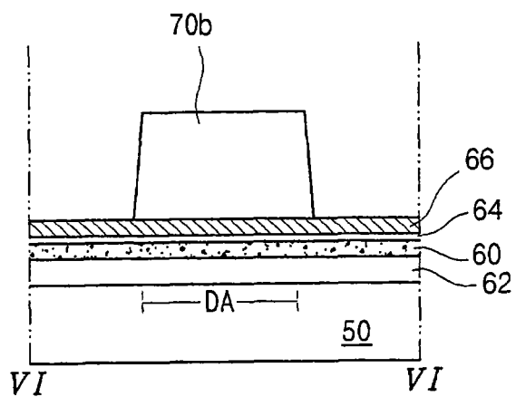
图 6C 现有技术
