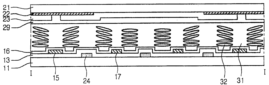
图 2 现有技术
