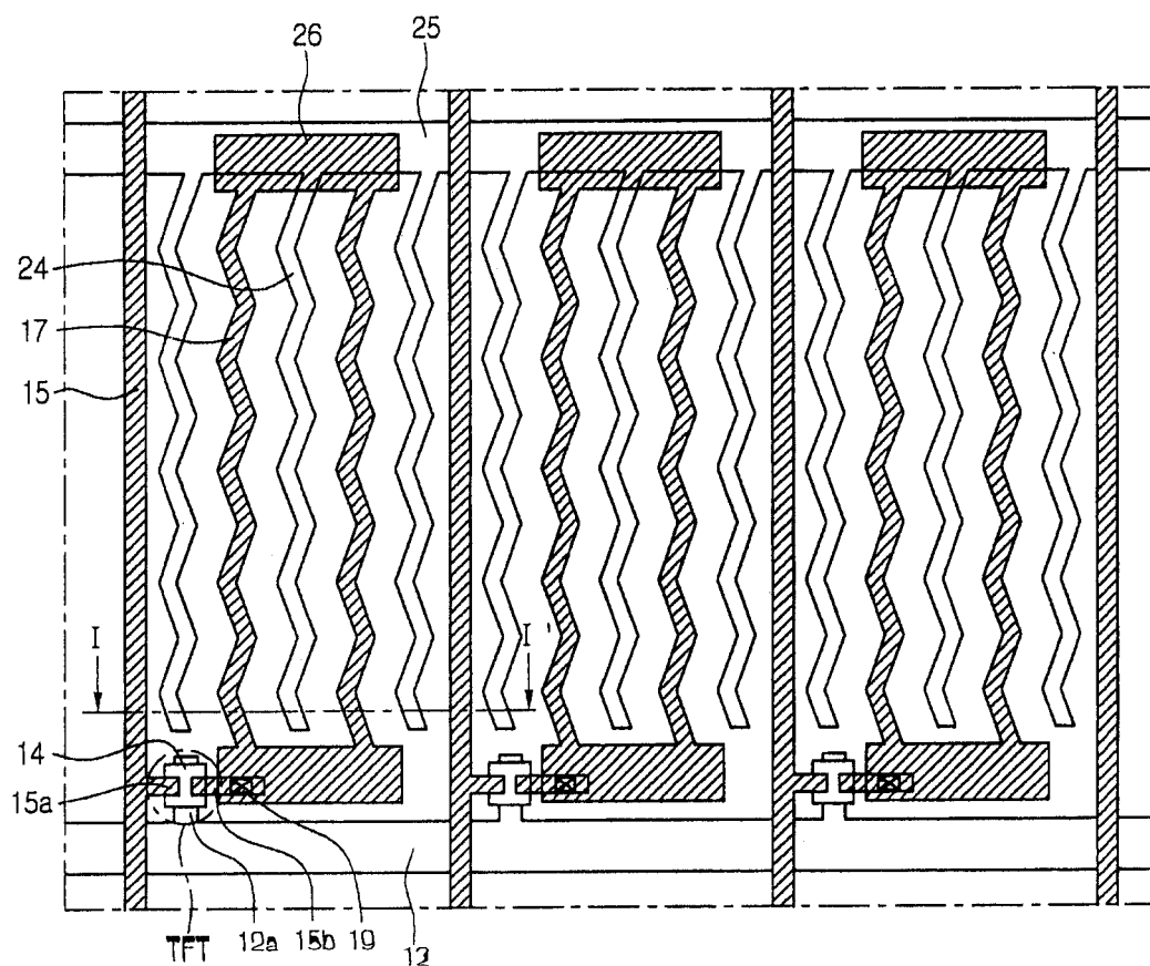
图 1 现有技术
