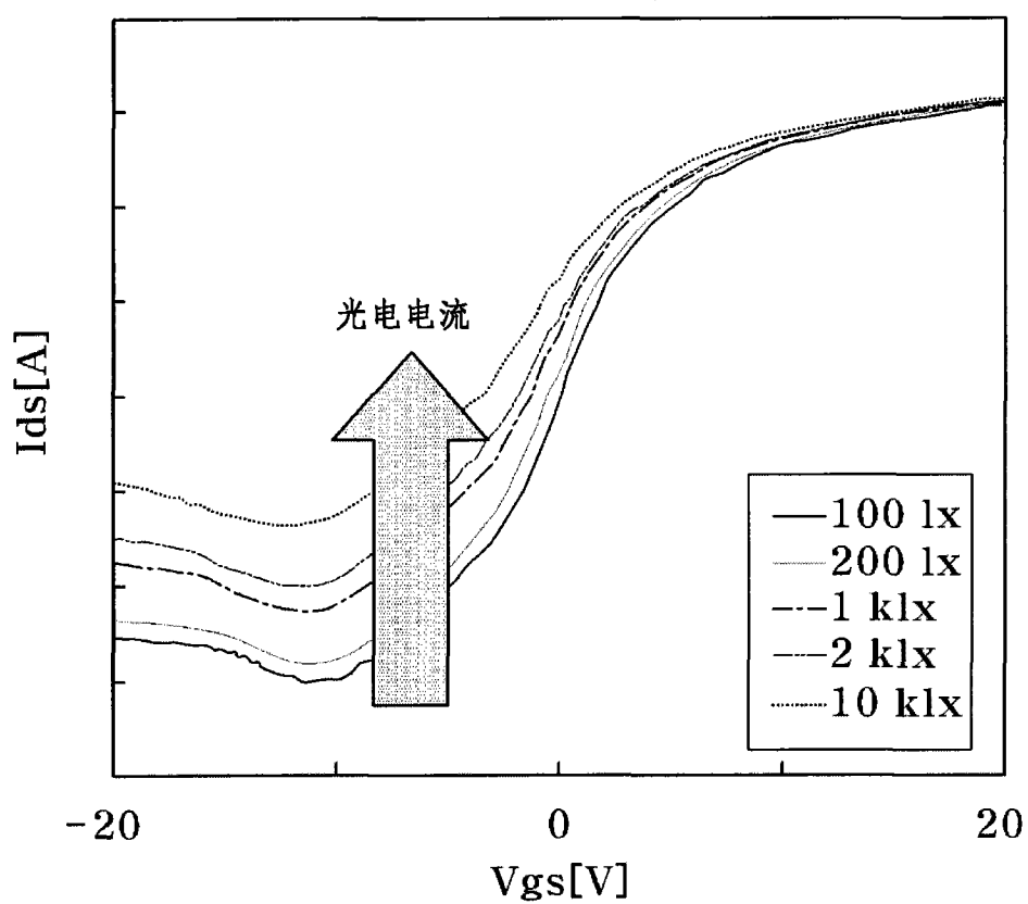
根据照度的变化曲线 ( V_{ds}=5V )
