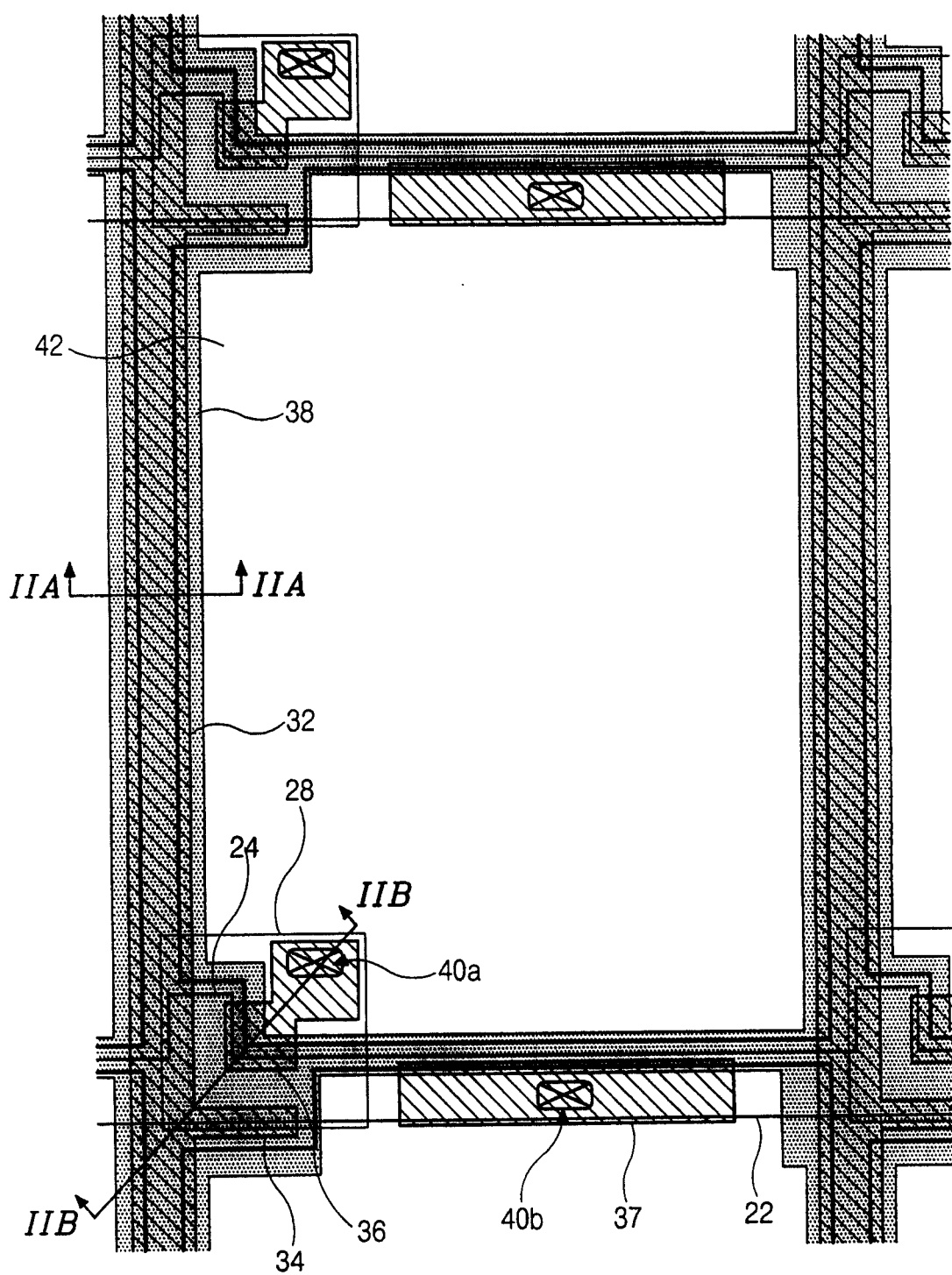
图 1 现有技术
