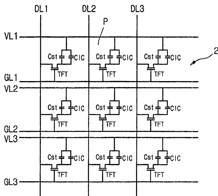
图 1 现有技术
