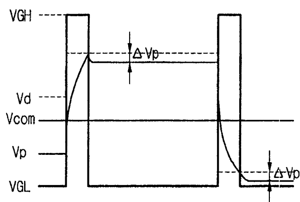
图 2 现有技术
