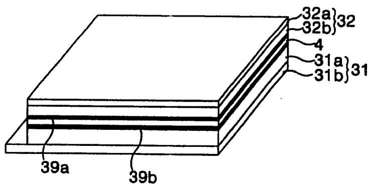
图 2 现有技术
