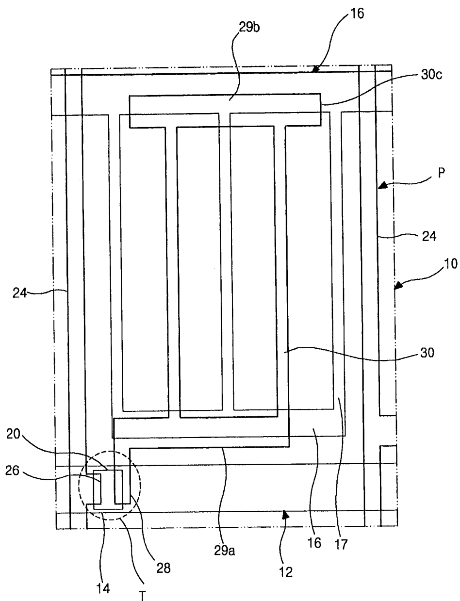
图 3 现有技术
