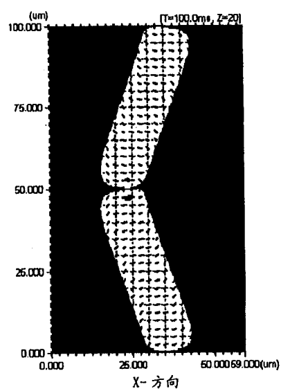
图 5 现有技术
